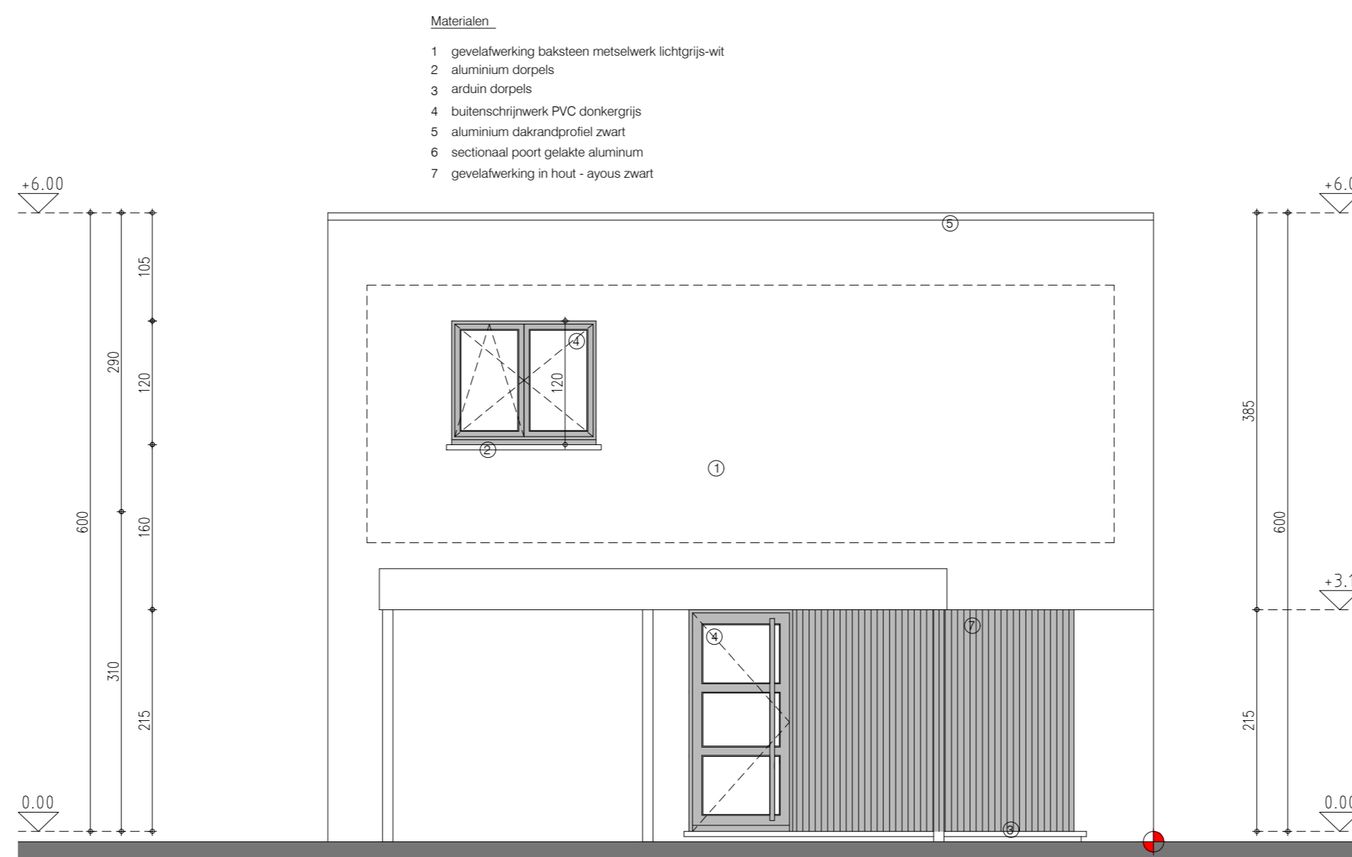
gevel noord - linker zijgevel lot 39
