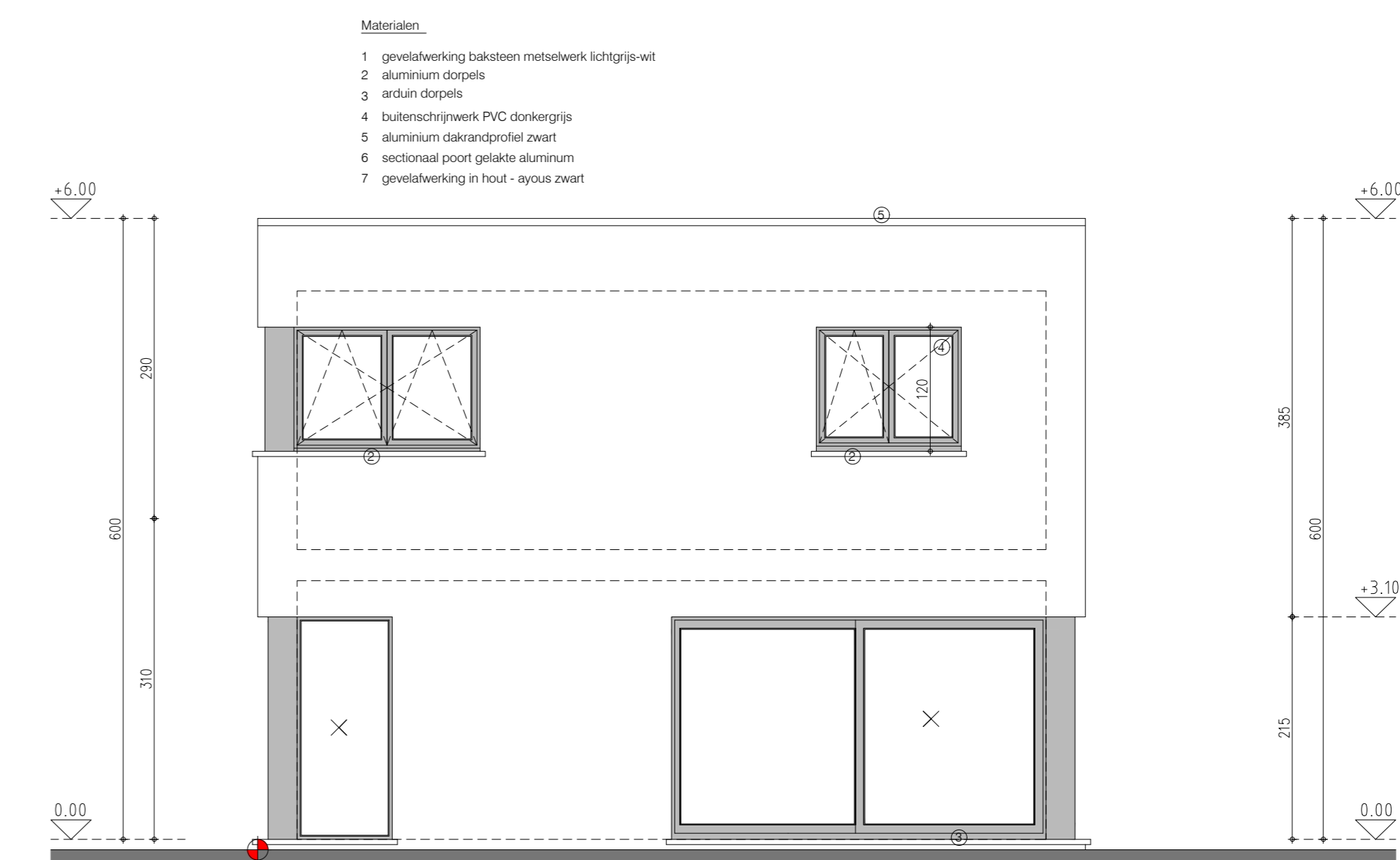
gevel zuid - rechter zijgevel lot 39
