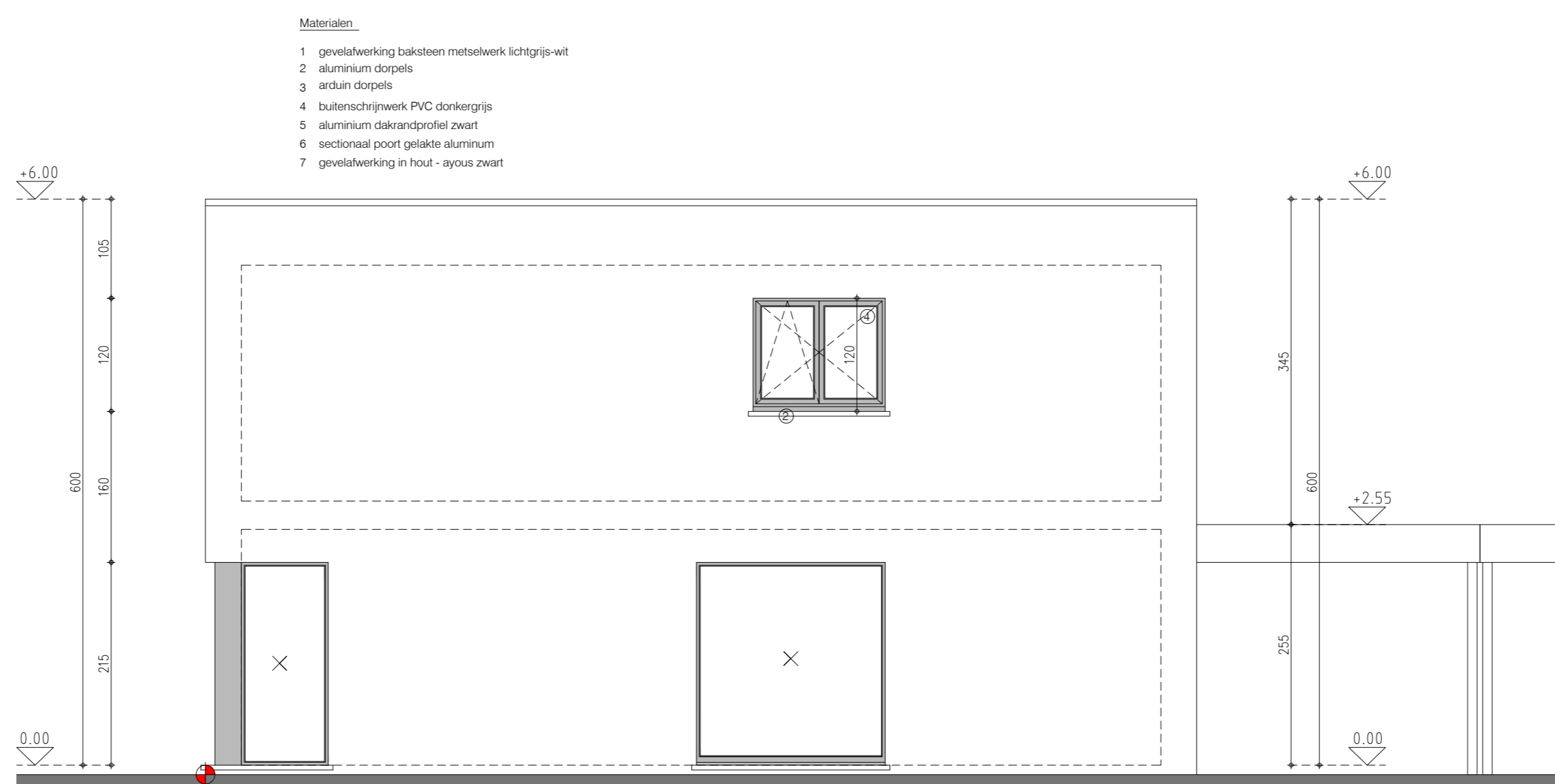
gevel oost - achtergevel lot 39
