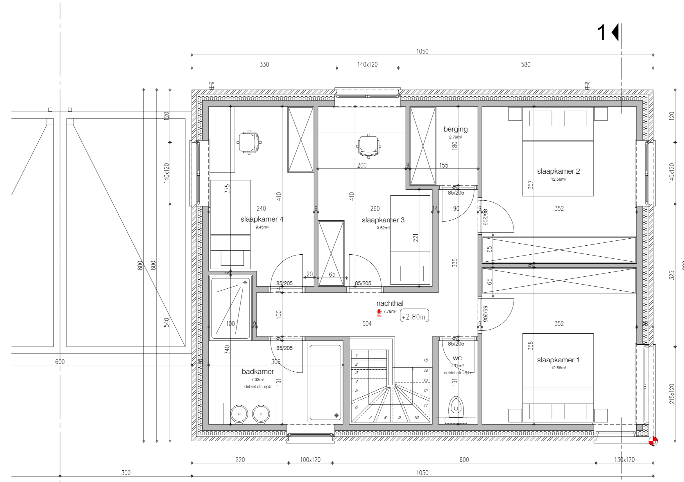
verdiepingsplan lot 39 84.00 m 2 bruto opp. 70.51 m 2 netto opp.
