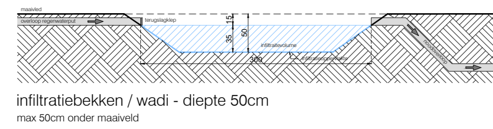
infiltratiebekken / wadi - diepte 50cm max 50cm onder maaiveld
