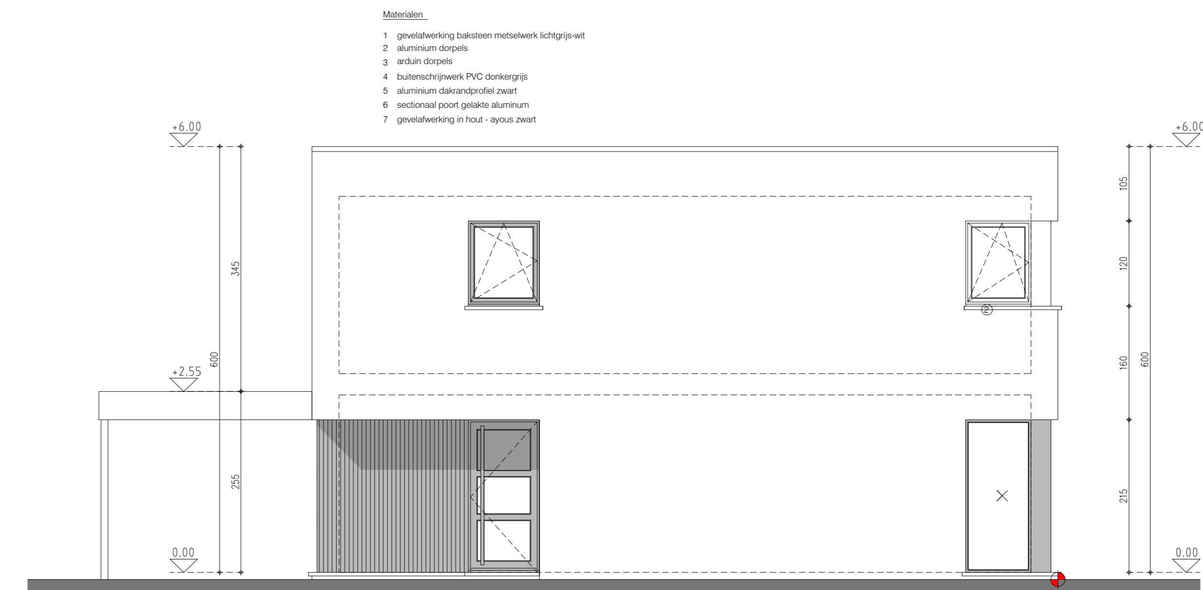
gevel west - voorgevel lot 39
