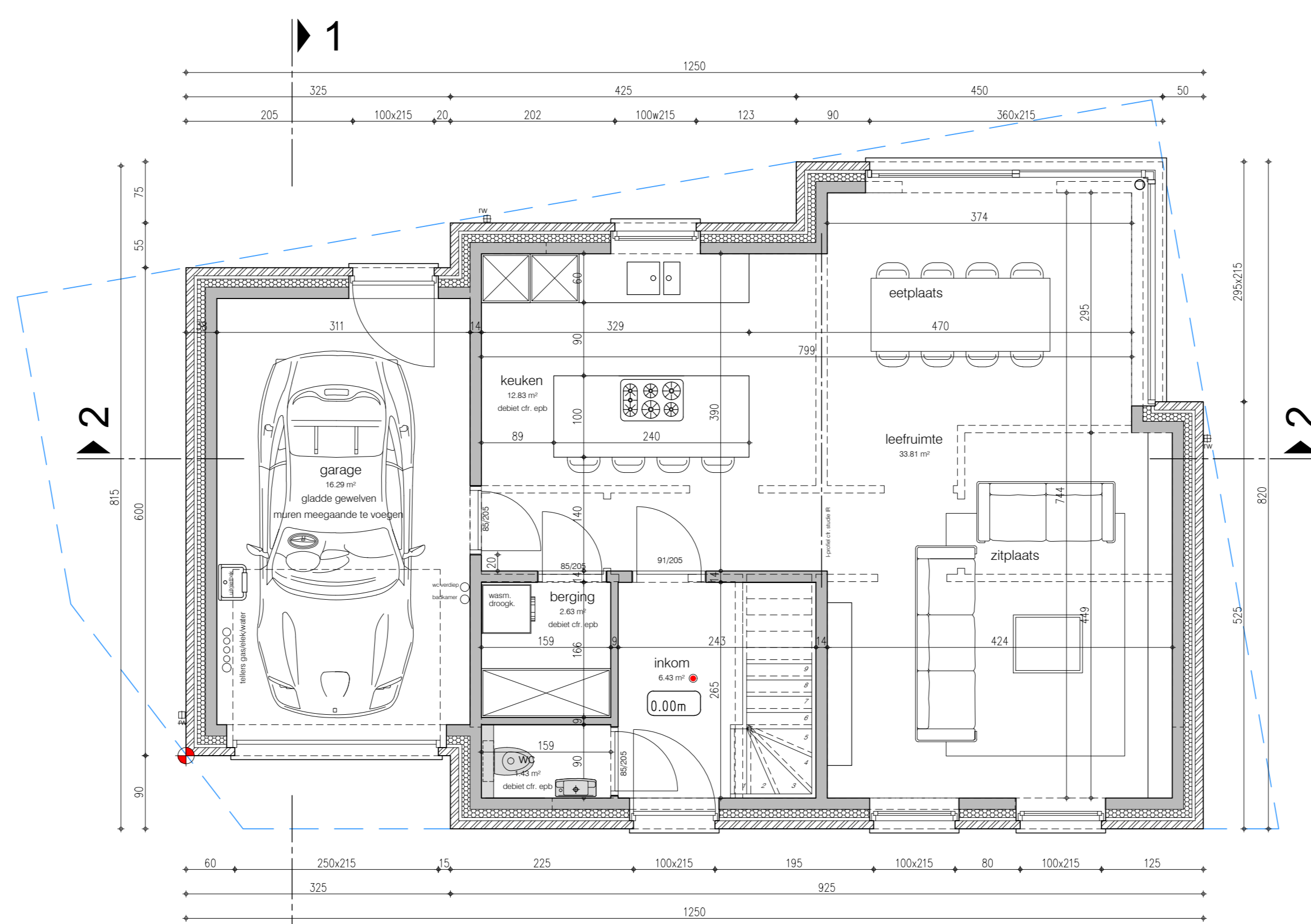
gelijkvloers lot 34 bruto opp. 90.68 m 2
