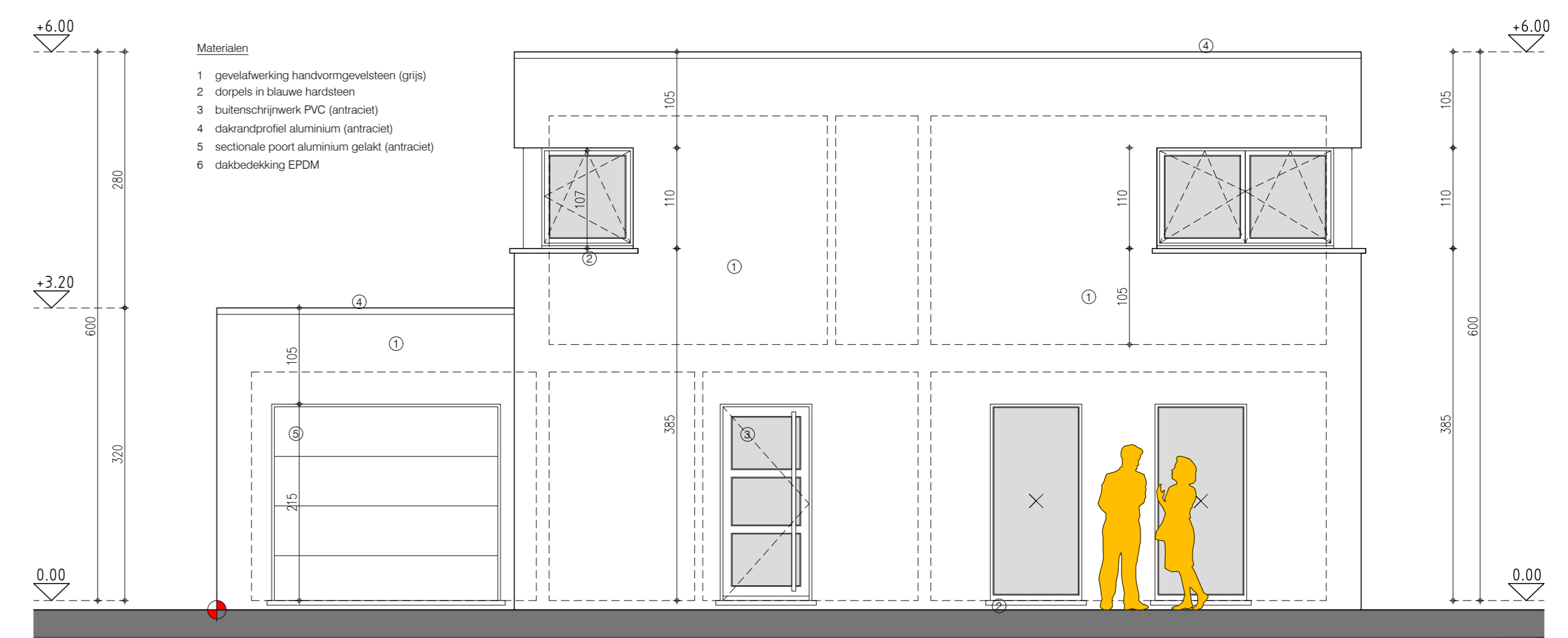
gevel noord - voorgevel lot 34
