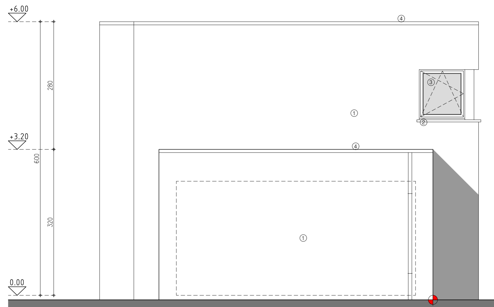
gevel oost - linker zijgevel lot 34
