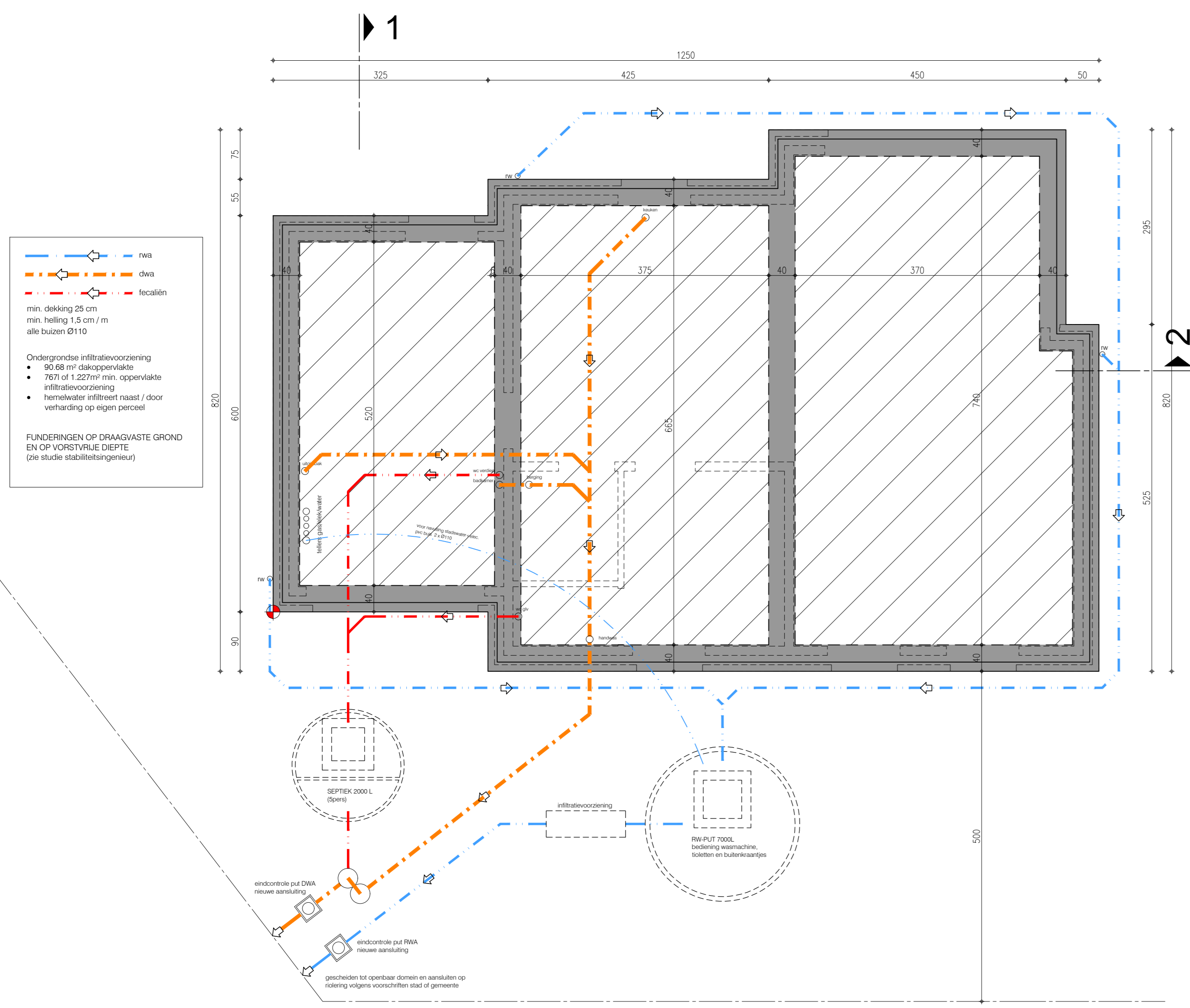
riolerings- en funderingsplan lot 34
