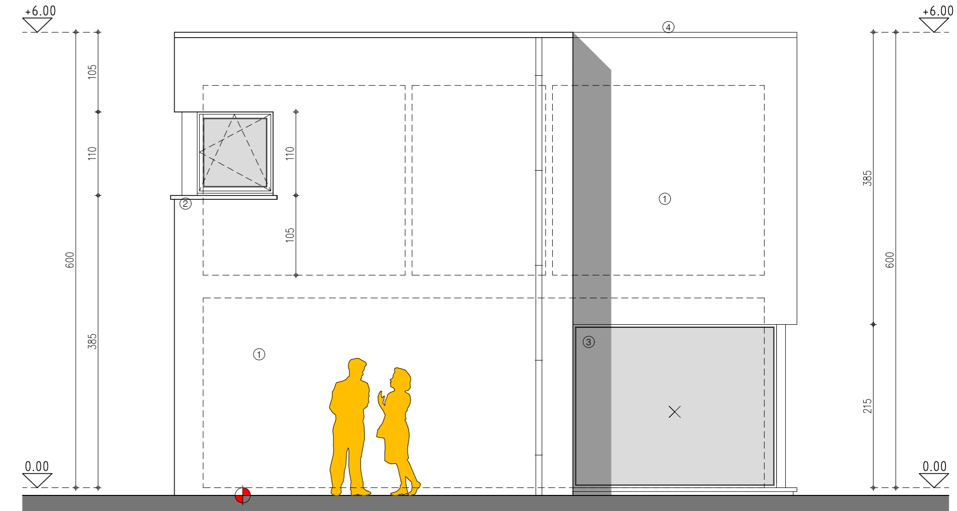
gevel west - rechter zijgevel lot 34
