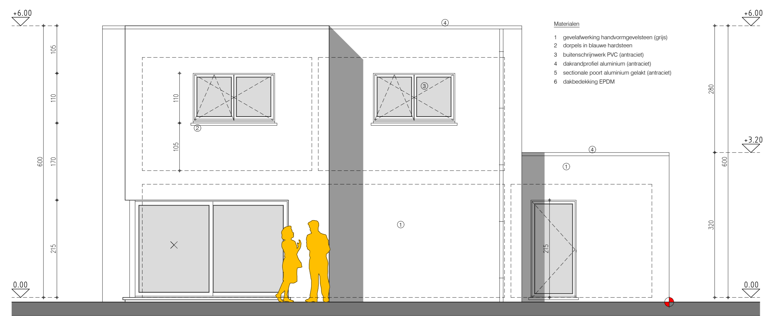
gevel zuid - voorgevel lot 34
