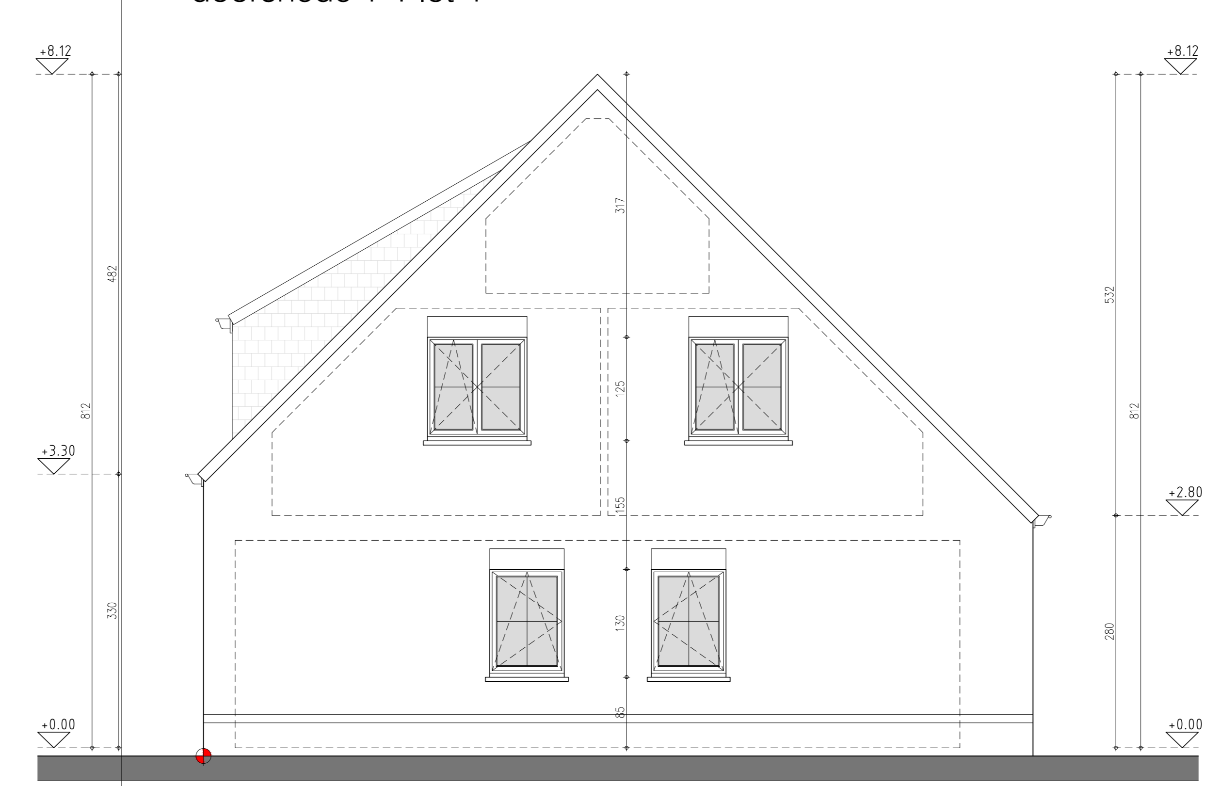
rechter zijgevel lot 4
