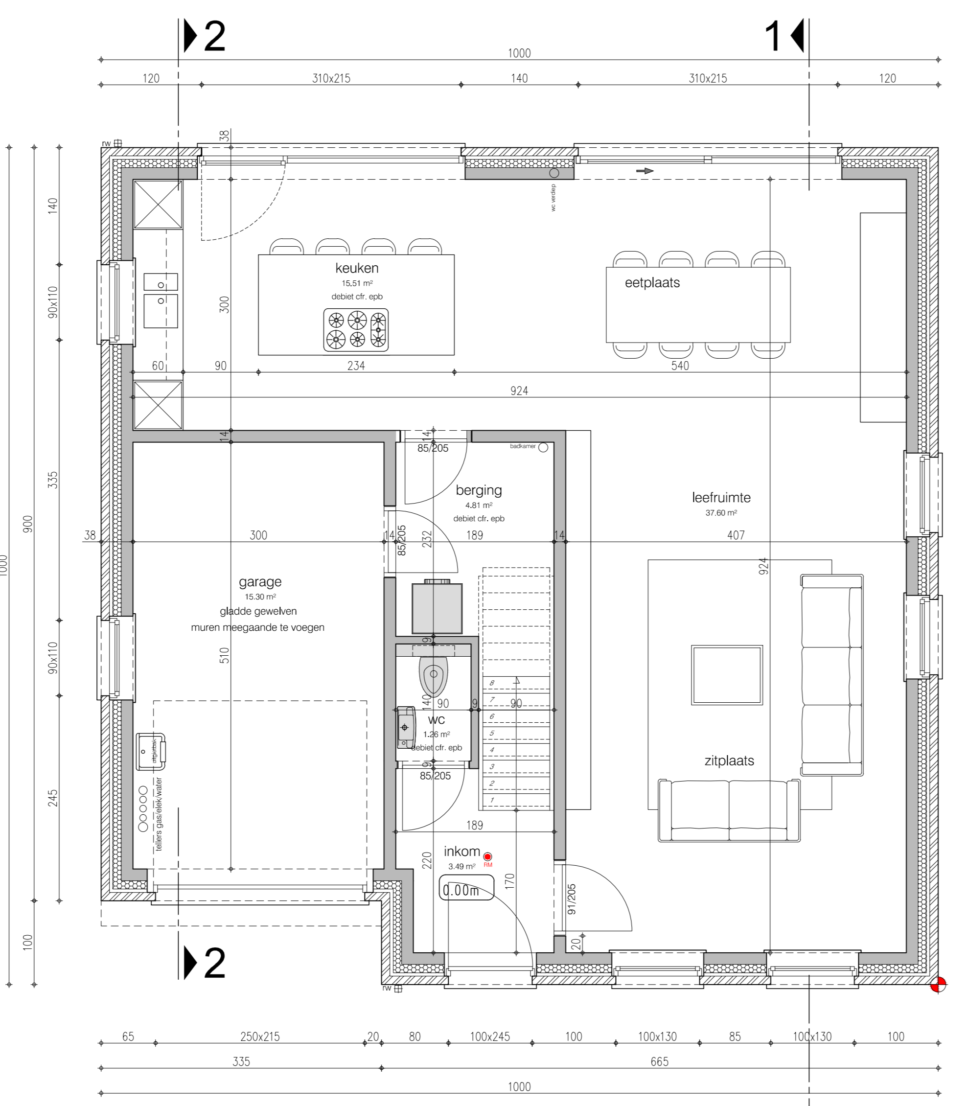
gelijkvloers lot 4 / 96.65 m² bruto opp.
