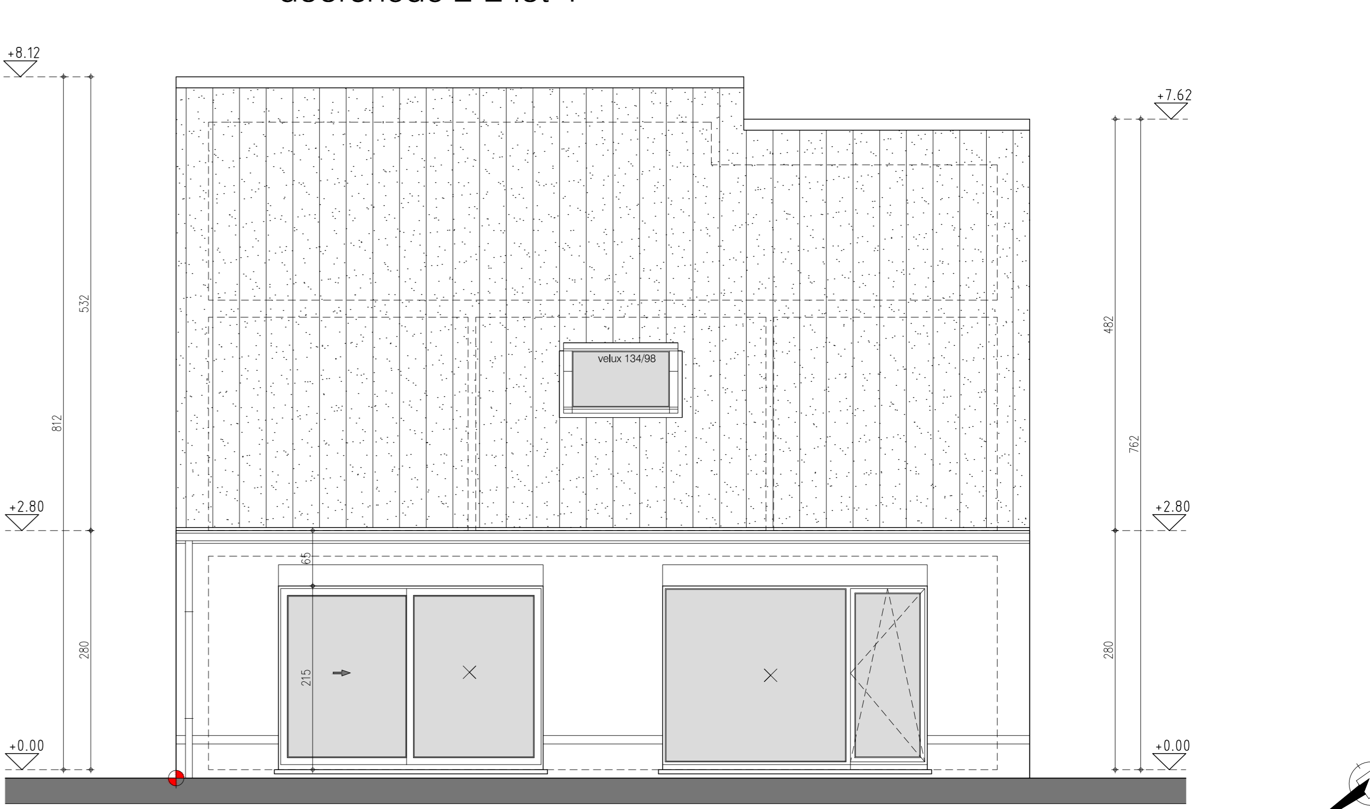
achtergevel lot 4
